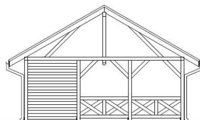
ELEWACJA WSCHODNIA skala 1:50
