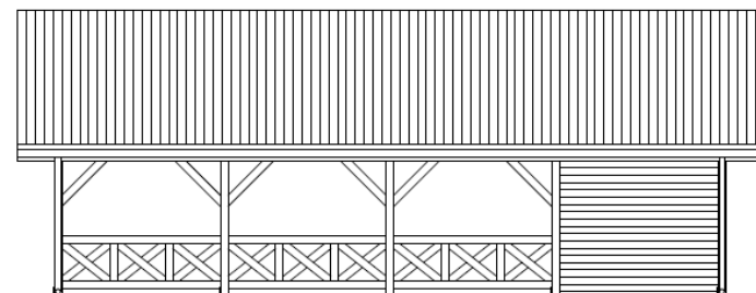
ELEWACJA POŁUDNIOWA skala 1:50
