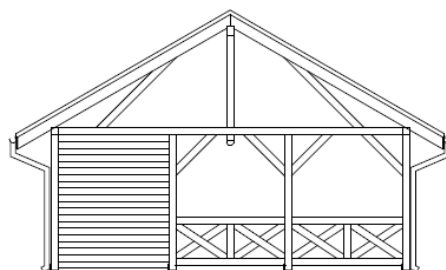
ELEWACJA WSCHODNIA skala 1:50
